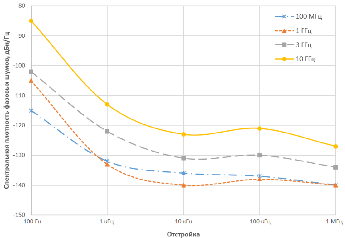
Типовой уровень фазовых шумов, MWR-ULPN
